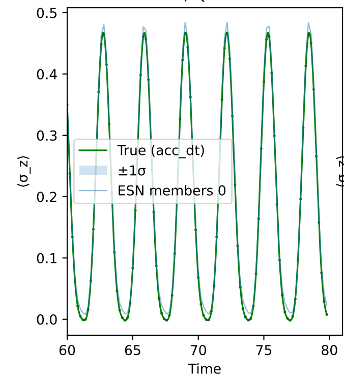
N=4, Qubit=2
