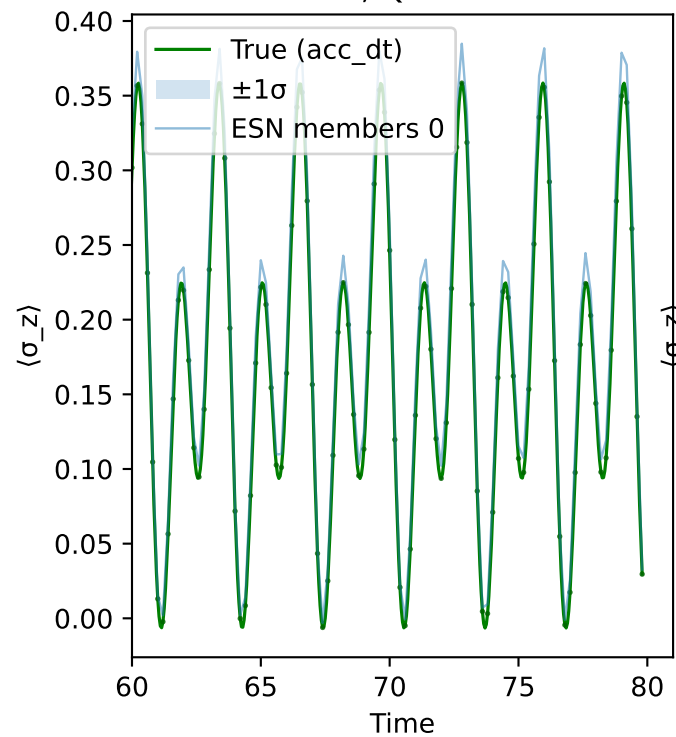
N=4, Qubit=3
