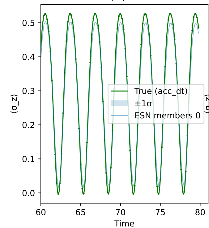
N=4, Qubit=3
